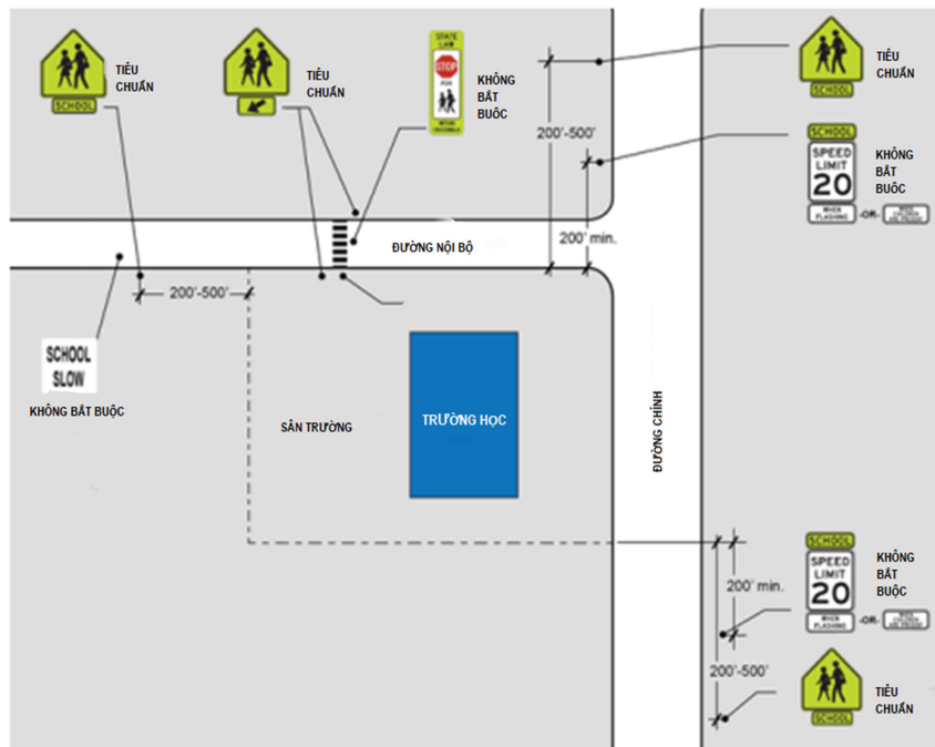
Hình 49. Mô hình bố trí hệ thống ATGT theo New Jersey School Zone
